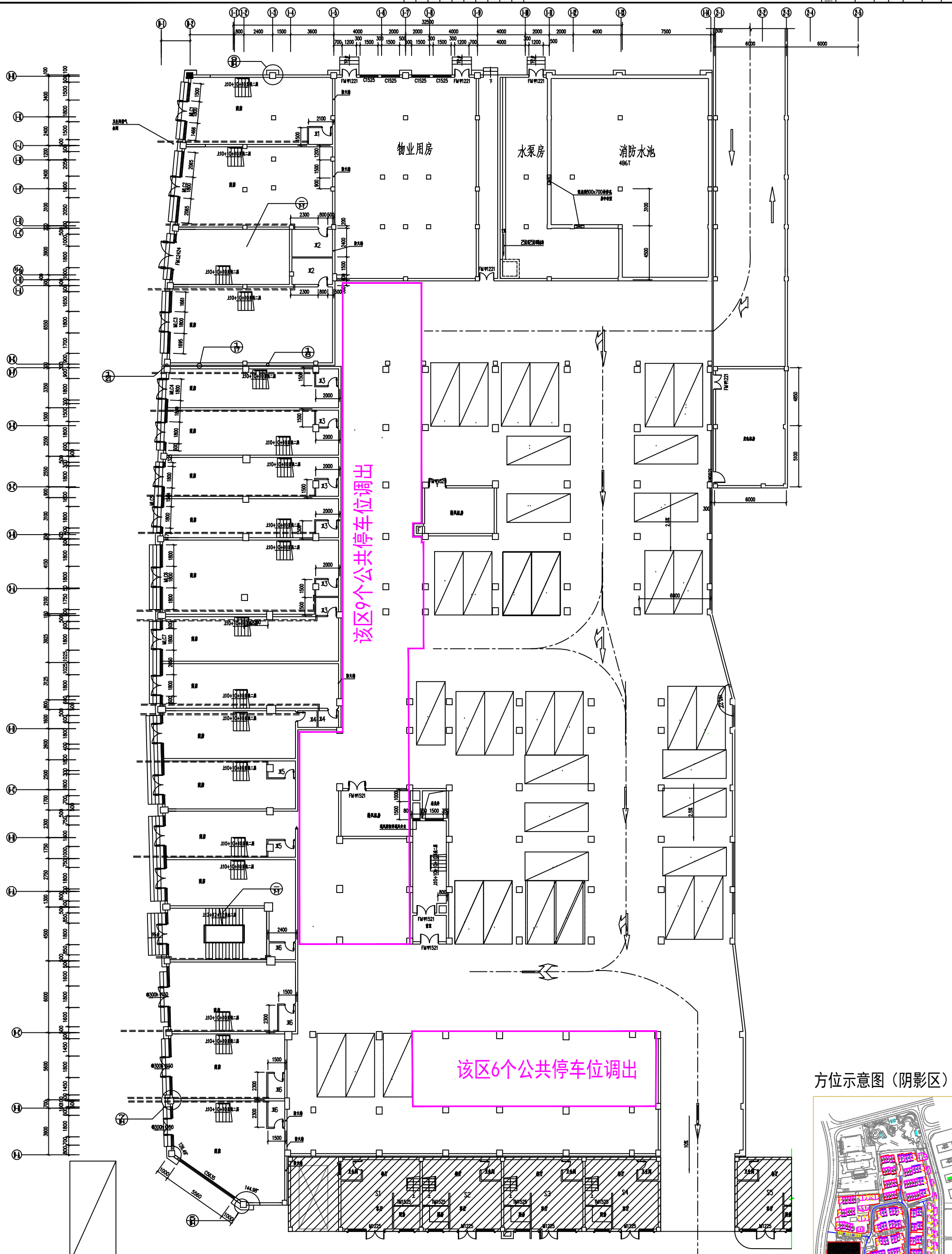
组团一地下三层(193.30标高层)车库局部调整后平面图
